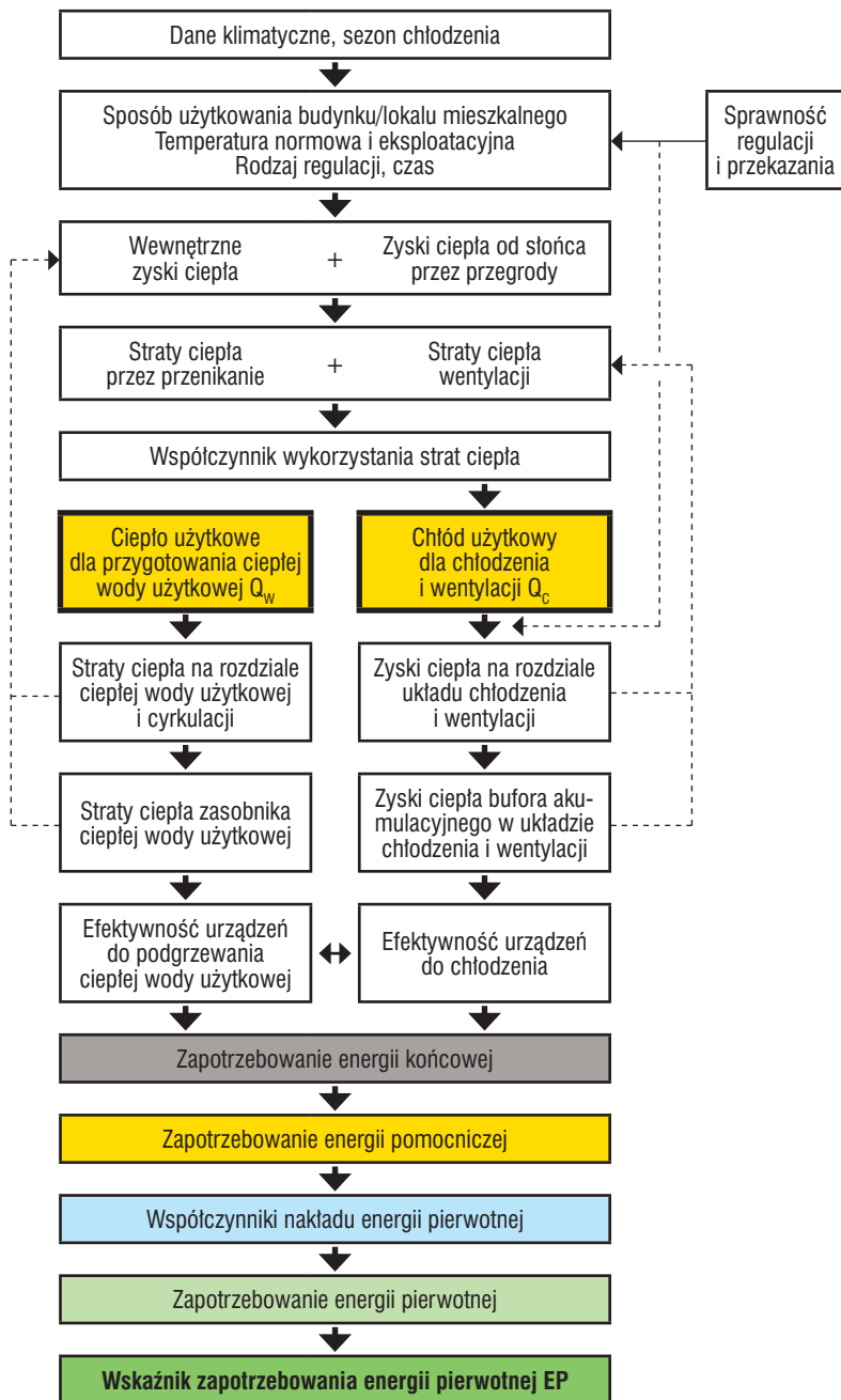
Rys. 1. Schemat blokowy obliczania wskaźnika zapotrzebowania na energię pierwotną do chłodzenia i przygotowania ciepłej wody użytkowej (w budynkach wyposażonych w instalację chłodzenia)
